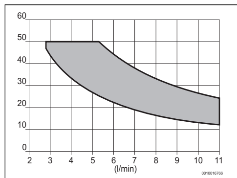
Fig. 25 Modelo 11 litros
