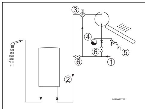
Fig. 12 Sistema solar
