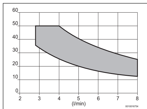
Fig. 24 Modelo 8 litros
