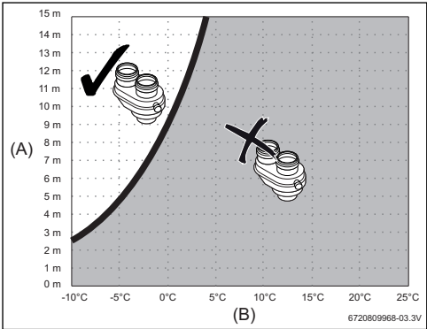
Fig. 10 Conductos separados
