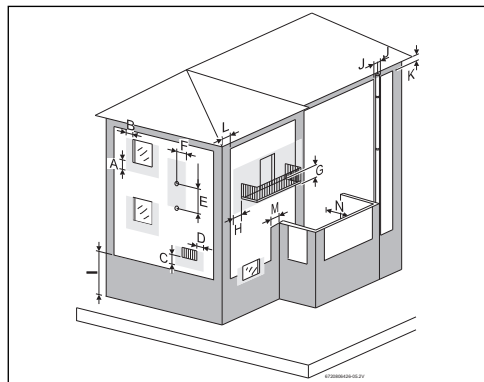
Fig. 14 Distancias mínimas a puntos de salida
