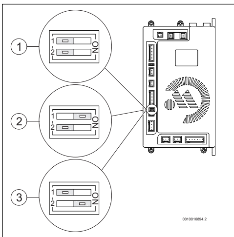
Fig. 16 Configuración de los interruptores
