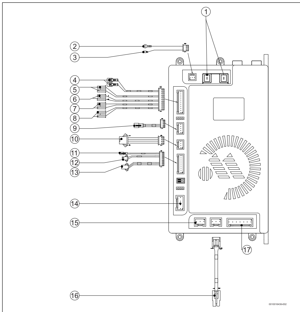
Fig. 23 Esquema de conexión
