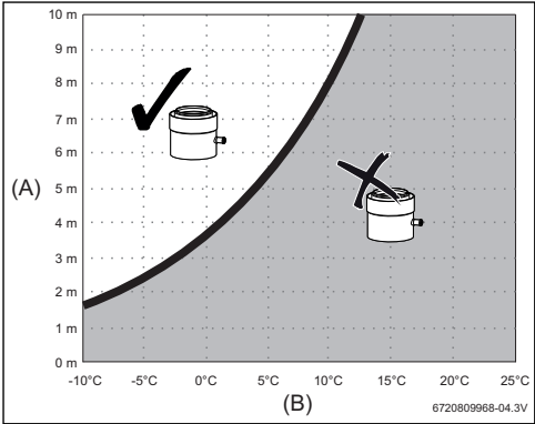
Fig. 9 Conductos concéntricos
