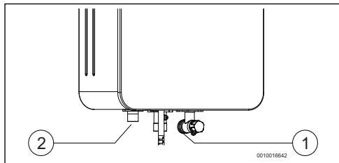
Fig. 15 Conexión de agua
