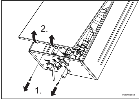
Fig. 21 Retirar la parte frontal
